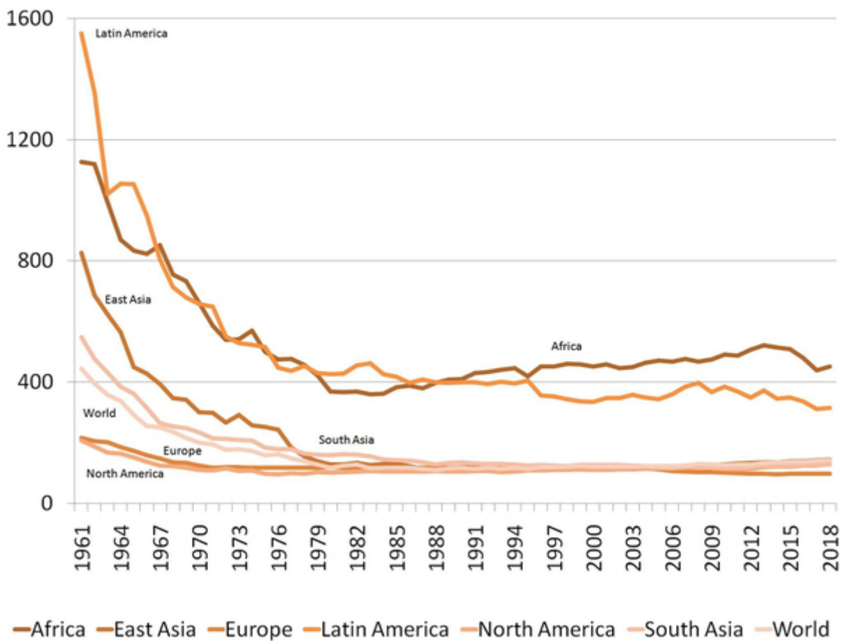
Graphique 2. Production agricole (tonnes) par unité d’engrais azoté de synthèse appliquée, de 1961 à 2018
